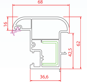
Hareketli Orta Kayıt
