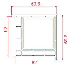
62x62 Kutu
