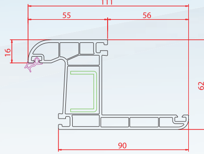
Super Pervazlı Kasa
