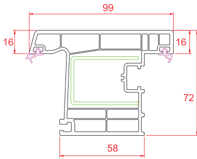
Dar Dışa Açılım Kapı Kanat
