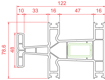
Kasa İçi Orta Kayıt
