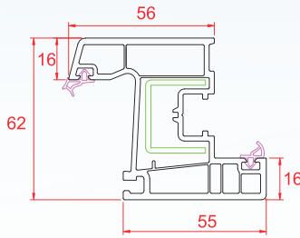
Pencere Kanat
