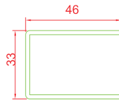
Dar Kapı Kanat Destek Sacı
