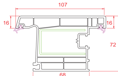
Dışa Açılım Kapı Kanat
