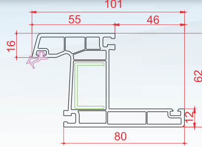
Pervazlı Kasa
