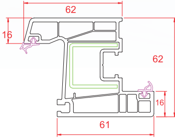
Süper Pencere Kanat
