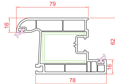
Dar Kapı Kanat
