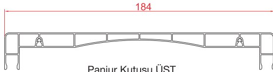
Panjur Kutusu ÜST
