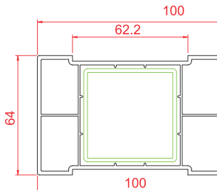
62x100 Kutu
