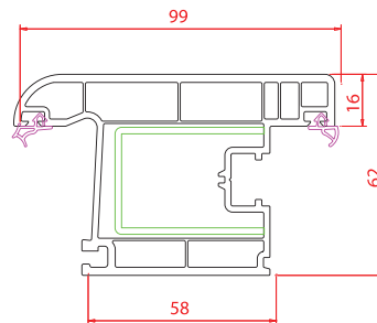
Dar Dış Açılım Kapı Kanat
