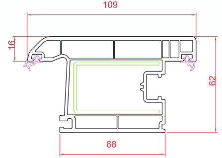
Dışa Açılım Kapı Kanat
