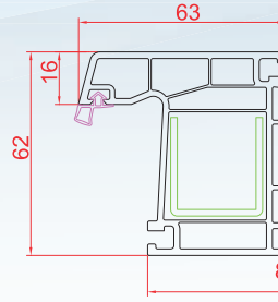
Geniş Pervazlı Kasa
