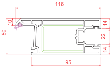
Kapı Kanat
