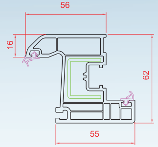
Pencere Kanat
