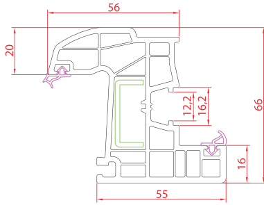
Pencere Kanat
