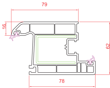
Dar Kapı Kanat
