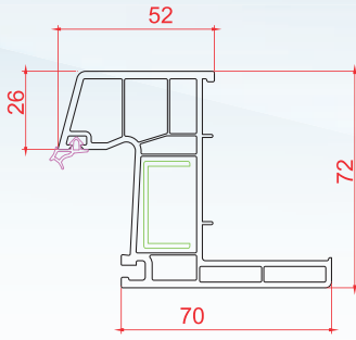
Pervazlı Kasa
