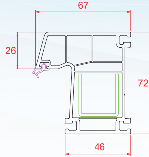
Süper Kasa
