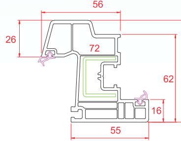
Damlalıklı Pencere Kanat
