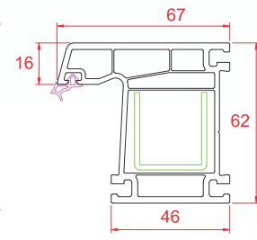
Süper Kasa
