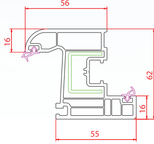
Pencere Kanat
