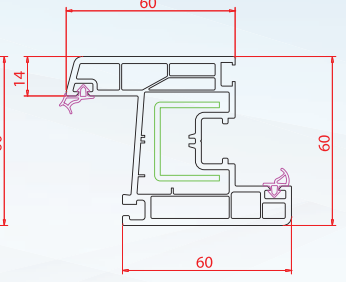
Pencere Kanat
