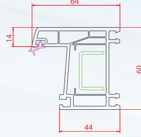
Kasa
