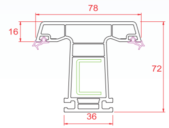
Dar Orta Kayıt
