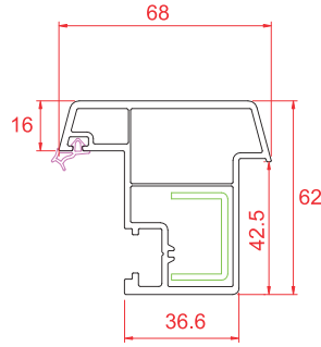
Hareketli Orta Kayıt
