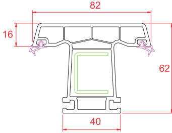
Orta Kayıt
