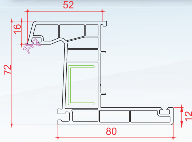
Süper Pervazlı Kasa
