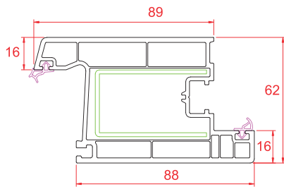
Kapı Kanat
