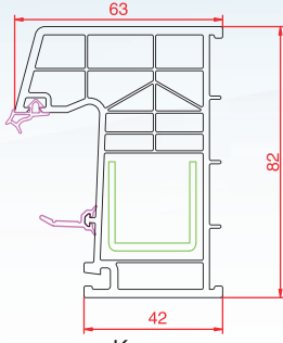
Kasa
