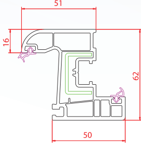
Dar Pencere Kanat
