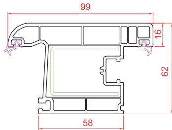
Dar Dışa Açılım Kapı Kanat
