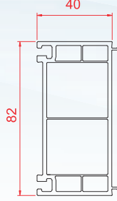
82 mm 4 cm Yükseltme
