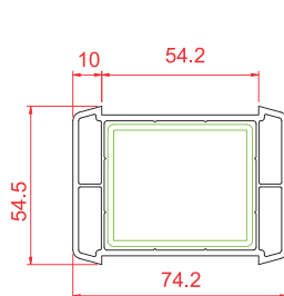
54x80 Kutu
