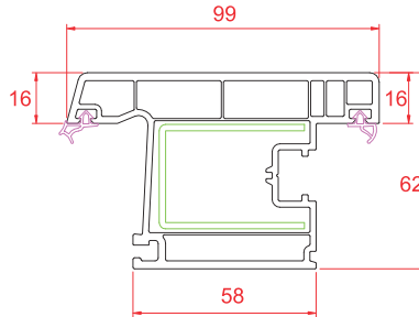
Dar Dışa Açılım Kapı Kanat
