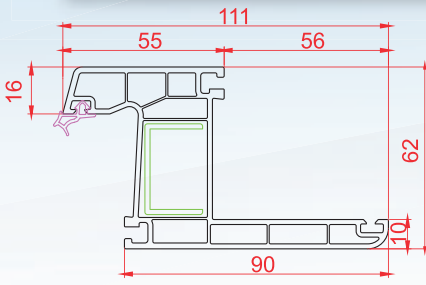
Süper Pervazlı Kasa
