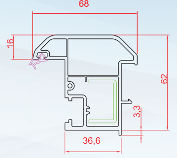
Hareketli Orta Kayıt
