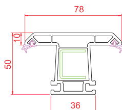
Orta Kayıt
