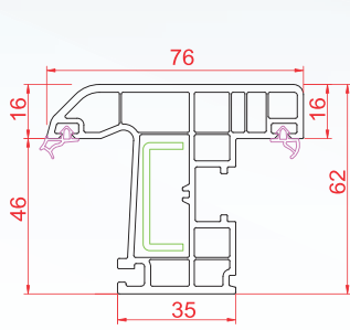
Dışa Açılım Pencere Kanat
