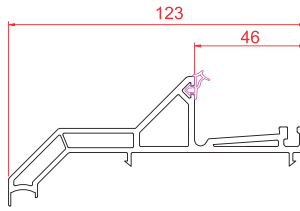
Kasa İçi Orta Kayıt Adaptörü
