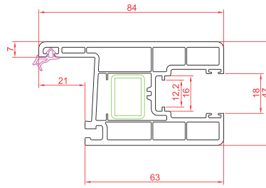
Pencere Kanat
