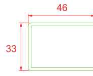
Dar Kapı Kanat Destek Sacı
