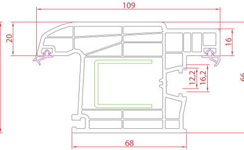
Dışa Açılım Kapı Kanat
