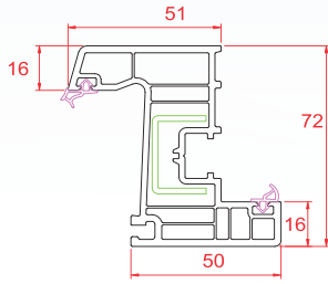
Dar Pencere Kanat
