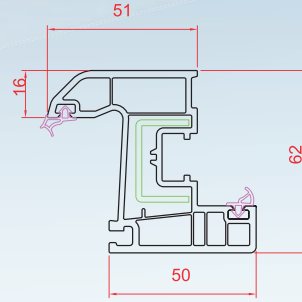
Dar Pencere Kanat
