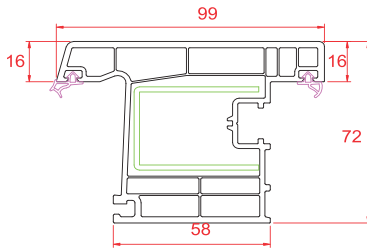
Dışa Açılım Dar Kapı Kanat
