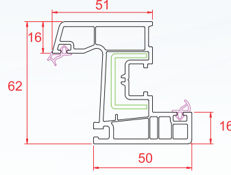
Dar Pencere Kanat
