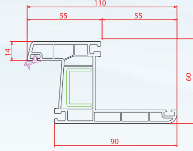
Pervazlı Kasa
