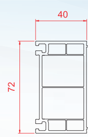
72 mm 4 cm Yükseltme
