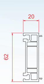
62 mm 2 cm Yükseltme
