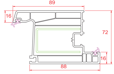
Kapı Kanat
