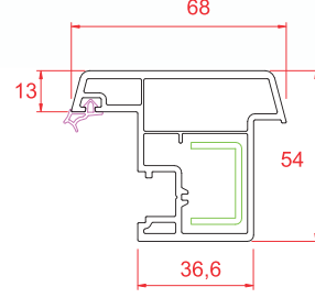
Hareketli Orta Kayıt
