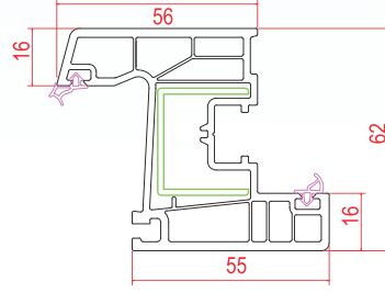
Pencere Kanat
