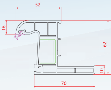
Pervazlı Kasa
