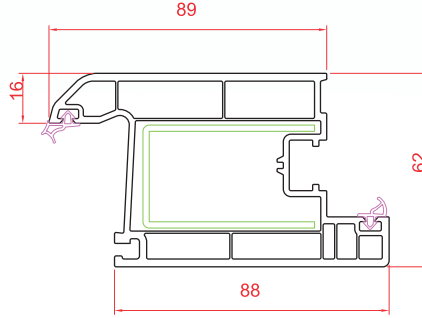
Kapı
