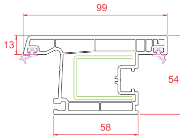
Dışa Açılım Kapı Kanat
