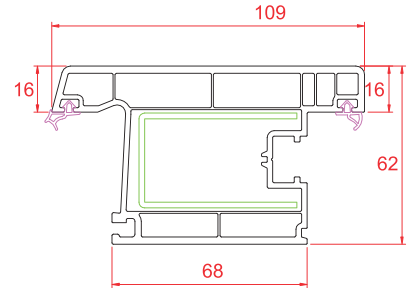
Dışa Açılım Kapı Kanat
