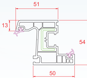
Dar Pencere Kanat
