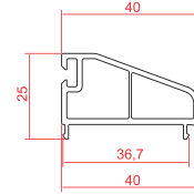
Yan Kapama
