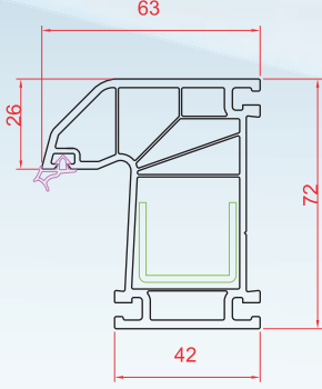
Kasa
