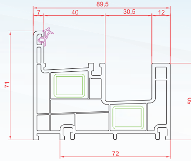
Tekli Kasa
