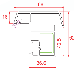
Hareketli Orta Kayıt
