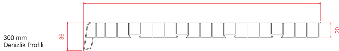
350 mm Denizlik Profili
