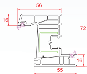
Pencere Kanat
