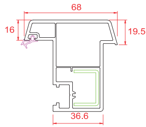
Hareketli Orta Kayıt
