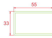
Kapı Kanat Destek Sacı
