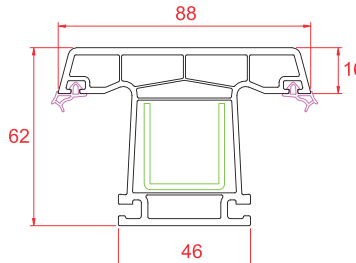
Süper Orta Kayıt
