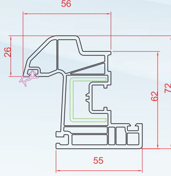
Damlalıklı Kanat
