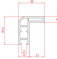
Sineklik Adaptörü
