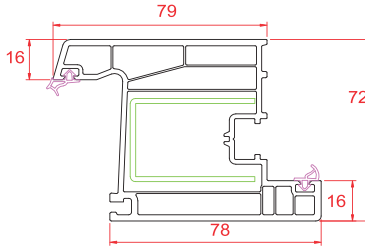
Dar Kapı Kanat
