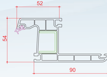
Süper Pervazlı Kasa
