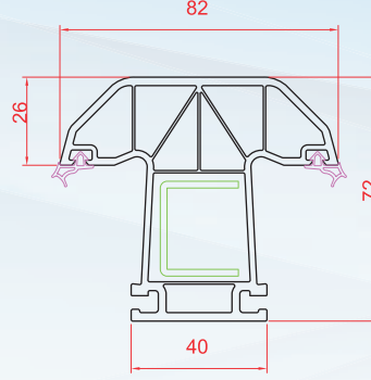
Orta Kayıt
