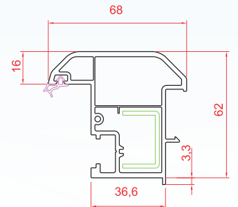
Hareketli Orta Kayıt
