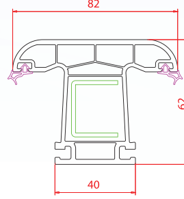
Orta Kayıt
