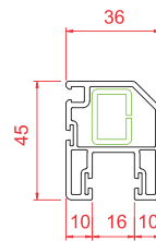
Sineklik
