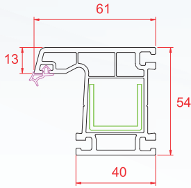
Kasa
