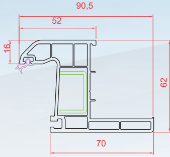
Pervazlı Kasa
