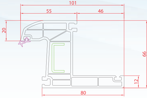
Pervazlı Kasa
